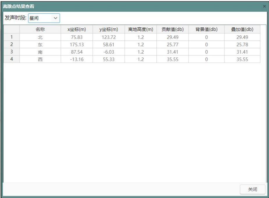
图 4-1 升压站厂界噪声预测结果模型截图（昼间）
