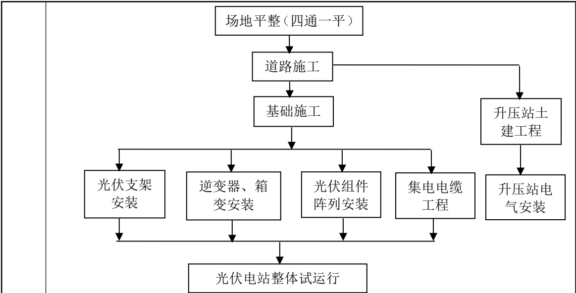
图 2-2 施工期工艺流程图
