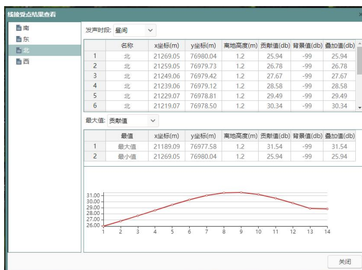
图 4-5 北厂界噪声预测结果模型截图（昼间）
