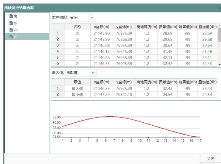
图 4-4 西厂界噪声预测结果模型截图（昼间）
