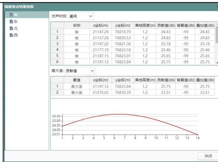
图 4-3 南厂界噪声预测结果模型截图（昼间）
