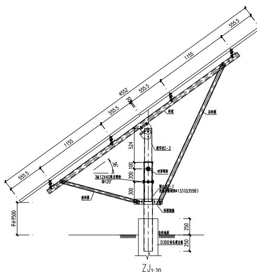
图 2-2 光伏支架方案
