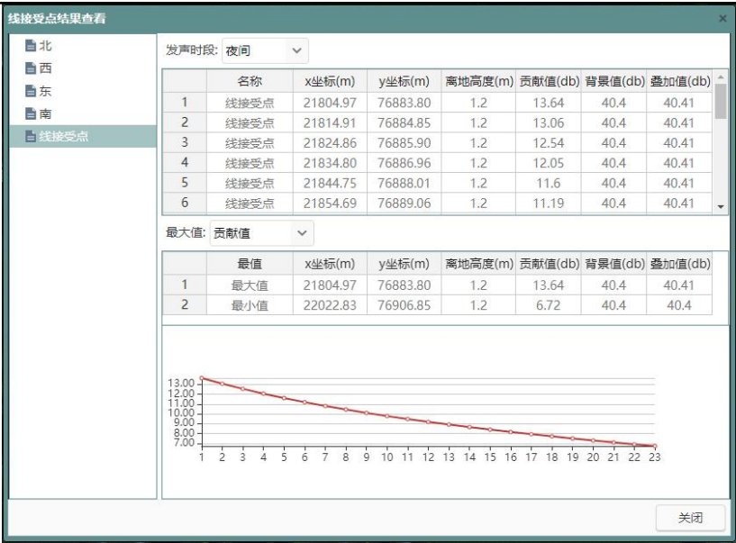
图 4-11 声环境保护目标噪声预测结果模型截图（夜间）
