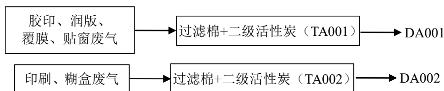
图 4-1 项目废气收集处理流程图
