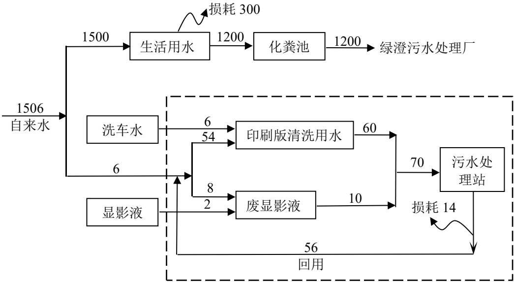
图 4-2 本项目水平衡图（单位：m³/a）
