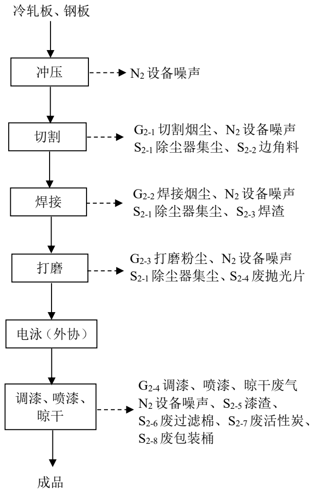
图2-2 汽车零部件生产工艺流程图
