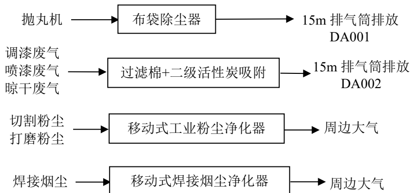
图 4-1 项目废气处理流程示意图
